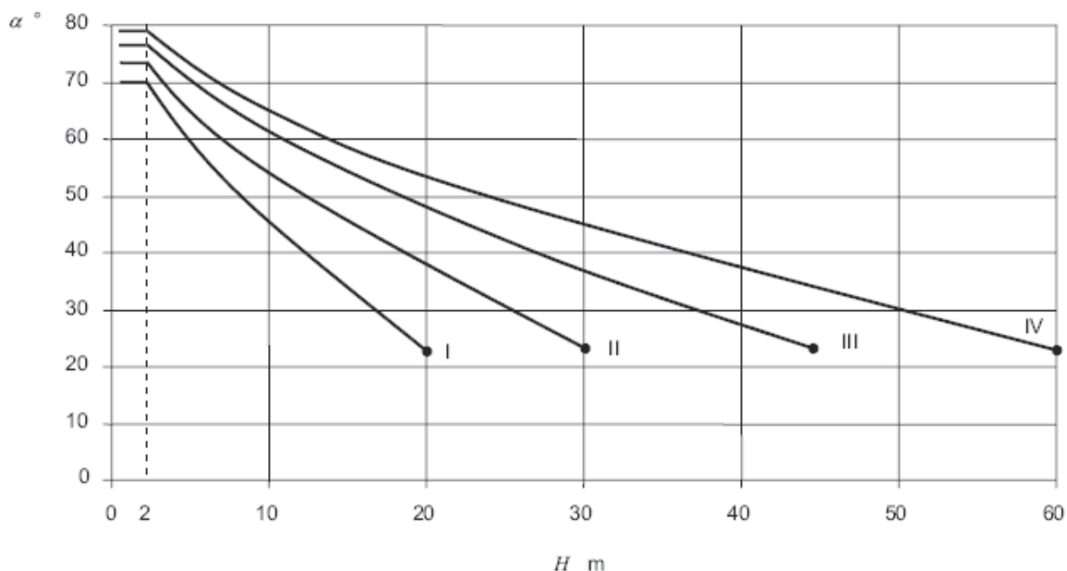
Фиг. 18. Стойности на мълниезащитния ъгъл \alpha в зависимост от нивото на мълниезащита и отстоянието H на върха на мълниеприемника от защитаваната хоризонтална повърхност
