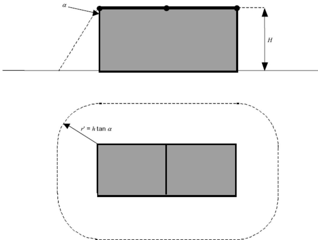
Фиг. 27. Защитна зона на прилежащо пространство, определяна по метода на мълниезащитния ъгъл, при мълниеприемна мрежа
