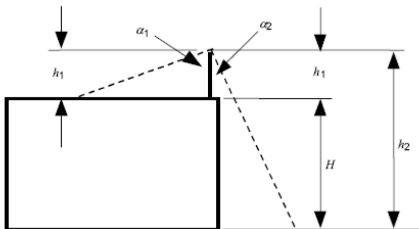
Фиг. 20. Мълниезащитна зона на вертикален прътов мълниеприемник
