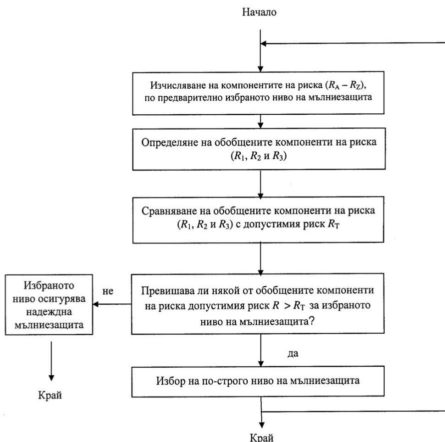
Фиг. 15. Алгоритъм за избор на ниво на мълниезащита
