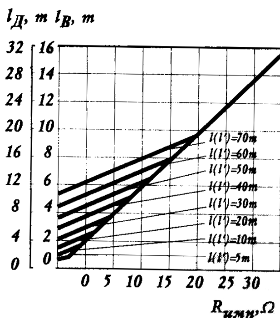
Фиг. 2. Мълниезащита чрез прътов мълниеотвод, изолиран от защитаваия обект
