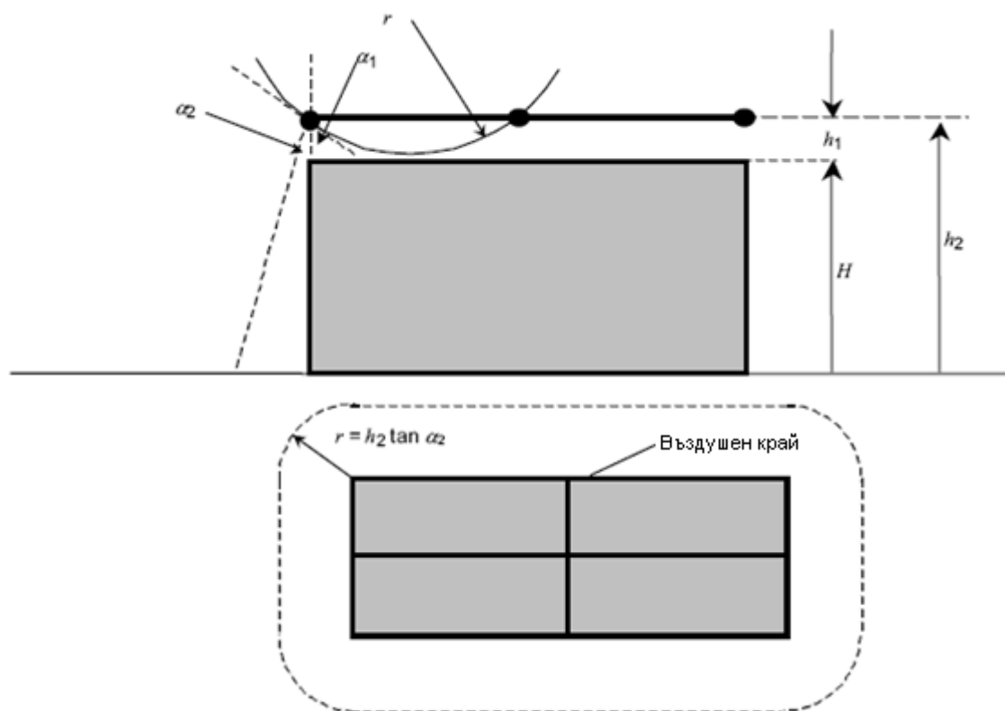
Фиг. 26. Защитна зона на прилежащо пространство, определяна по метода на фиктивната търкаляща се сфера, при мълниеприемна мрежа
