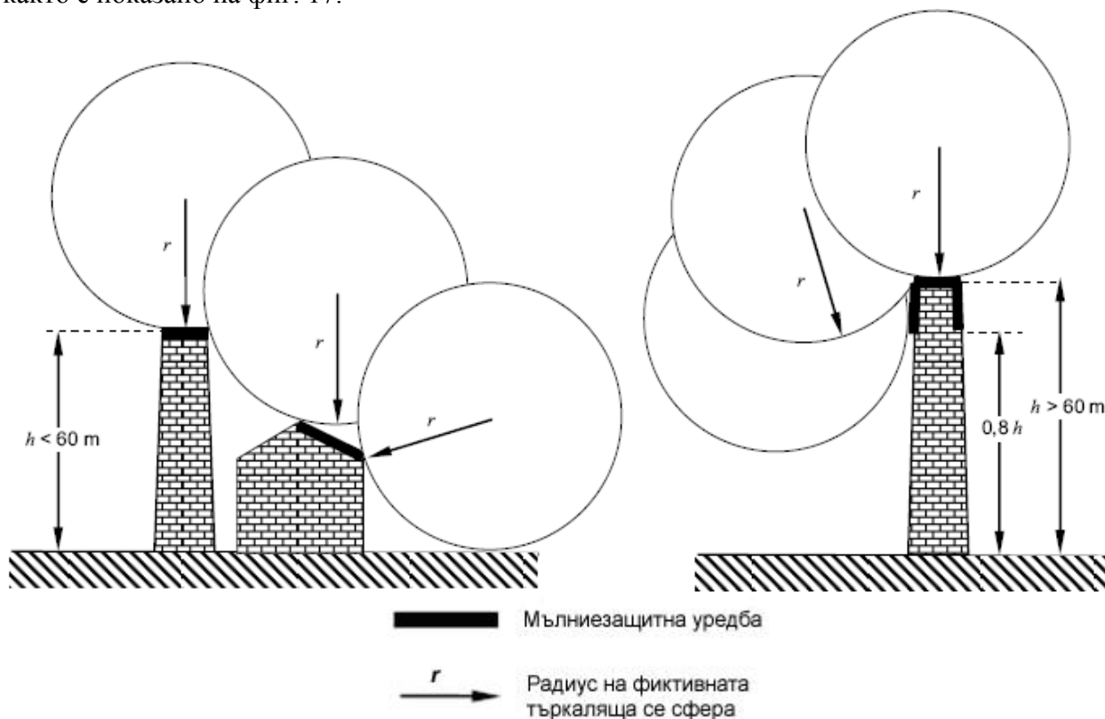
Фиг. 17. Определяне на мълниезащитната зона и проектиране на мълниеприемник/мълниеприемници по метода на фиктивната търкаляща се сфера
