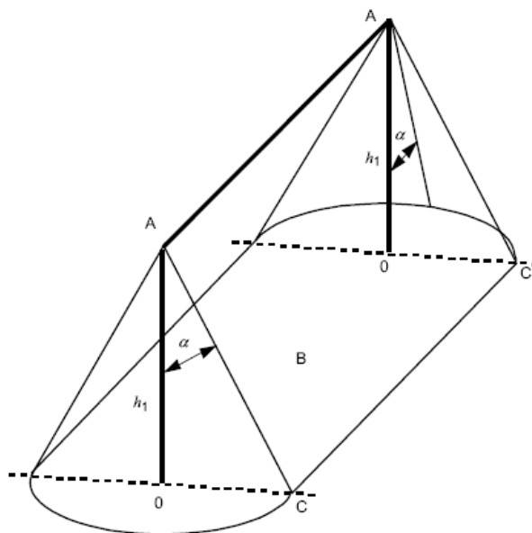
Фиг. 22. Мълниезащитна зона на мълниеприемен проводник между две мачти с равни височини
