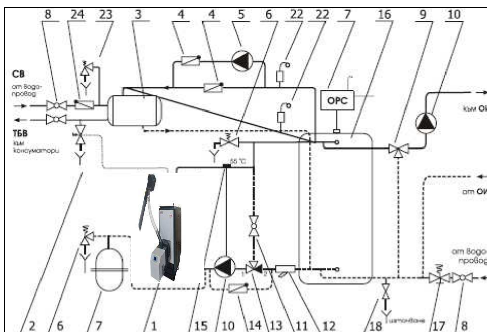
Фигура 16. Примерна принципна хидравлична схема за свързване на котел Bisolid Automat към отоплителна система
