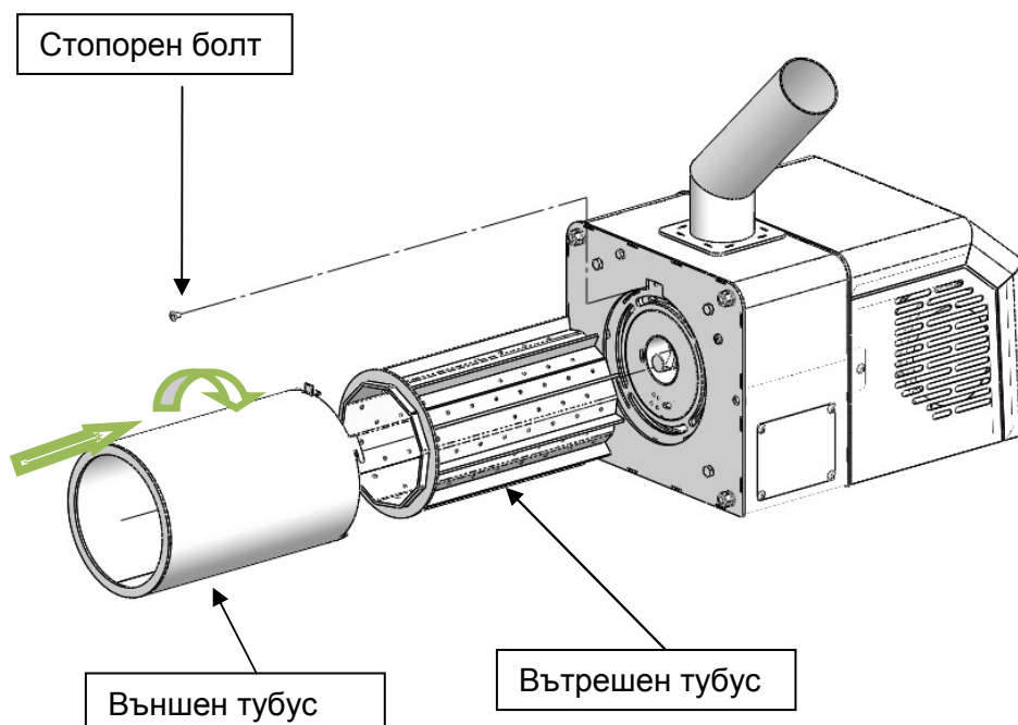
Фигура 17. Схема на основния модул на горелката с демонтиран тубус
