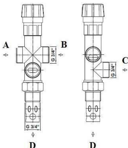
Фигура 25. Двупътен предпазен вентил DBV 1
