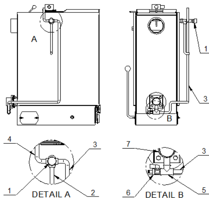
Фигура 26. Присъединяване на DBV 1 към котли Bisolid Automat
