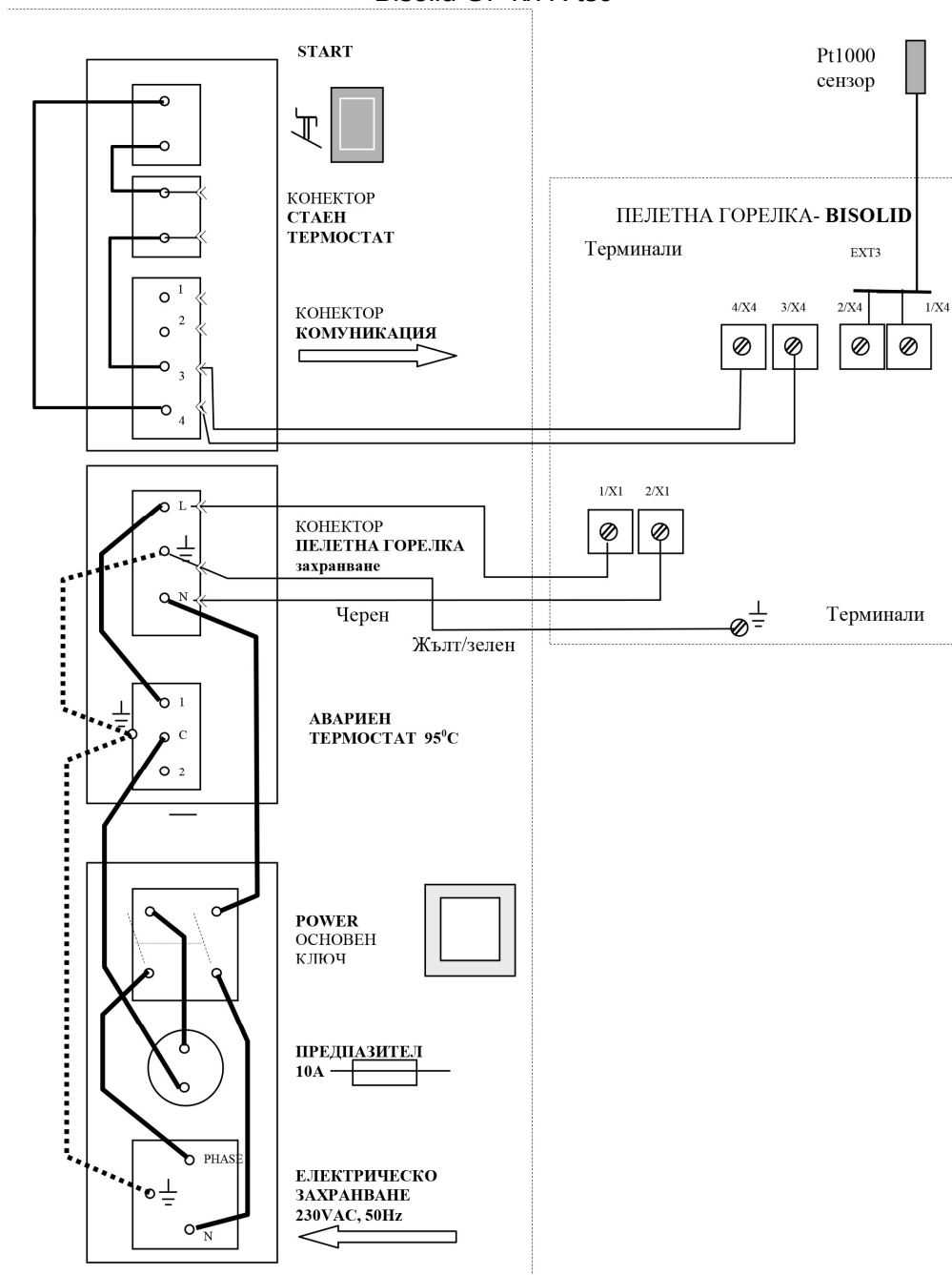
Фигура 22. Схема на панела с конектори за свързване на пелетната тубусна горелка Bisolid GP xx R tsc
