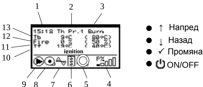
Фигура 20. Индикация на дисплея на пелетна горелка серия Bisolid GP xx R tsc
