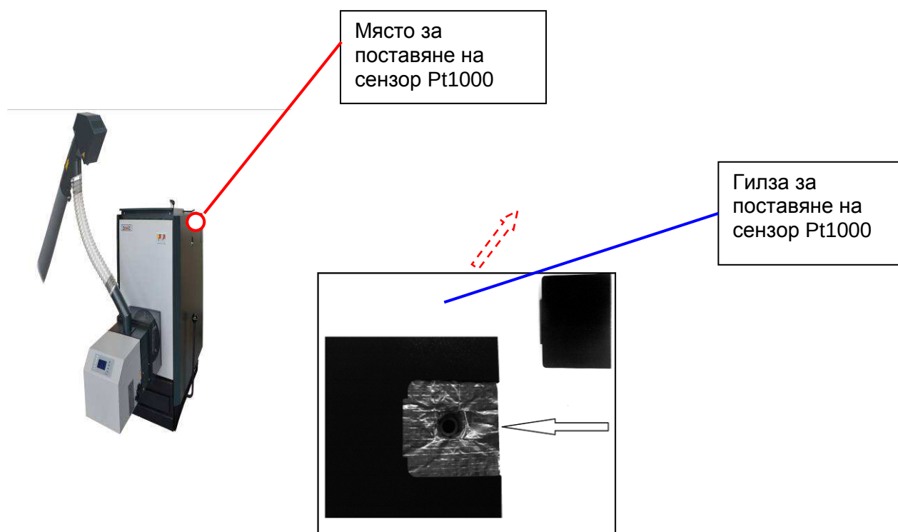
Фигура 23. Монтаж на сензора за температура на водата
