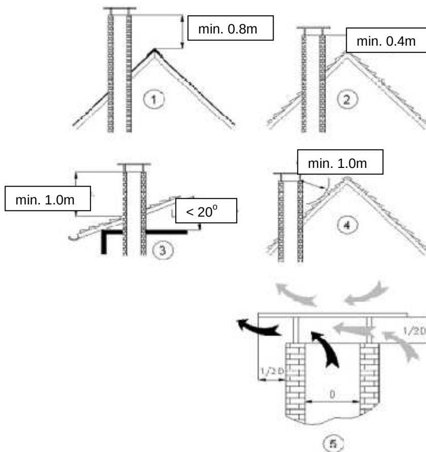
Фигура 30. Изисквания при изграждане на комина, над покрива на сградата
