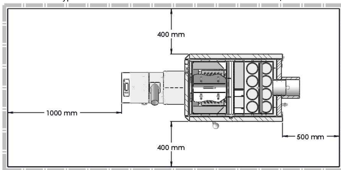
Фигура 24. Разположение на котела в котелното помещение
