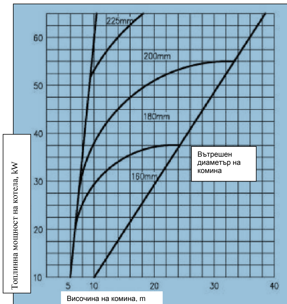
Фигура 29. Диаграма за оразмеряване на общата височина и минималния диаметър на комина
