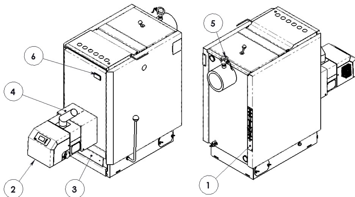
Фигура 6. Окомплектовка на котли серия Bisolid Automat
