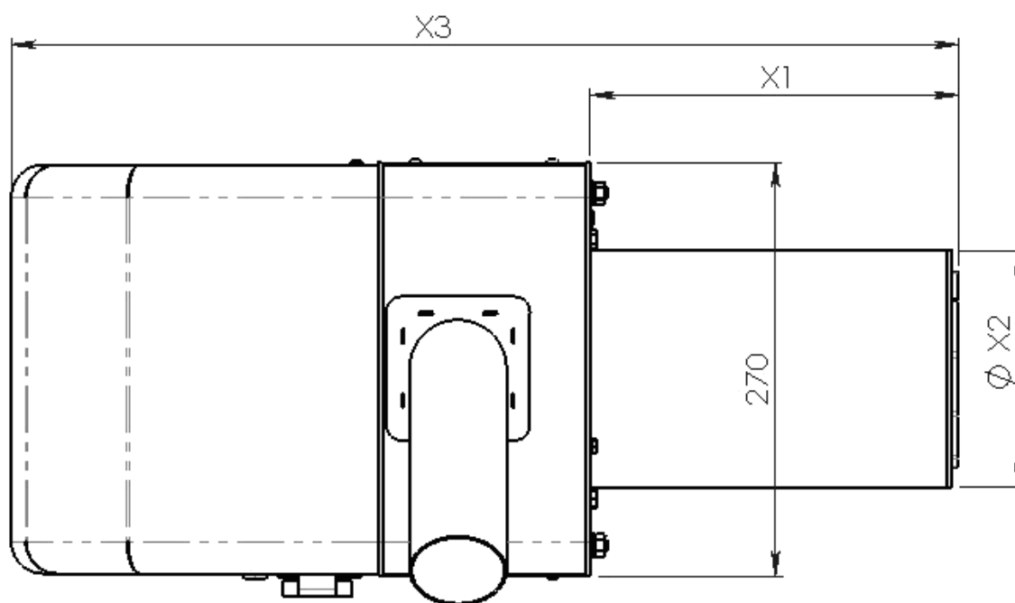
Фигура 15. Габаритни размери на основния модул на пелетната тубусна горелка
