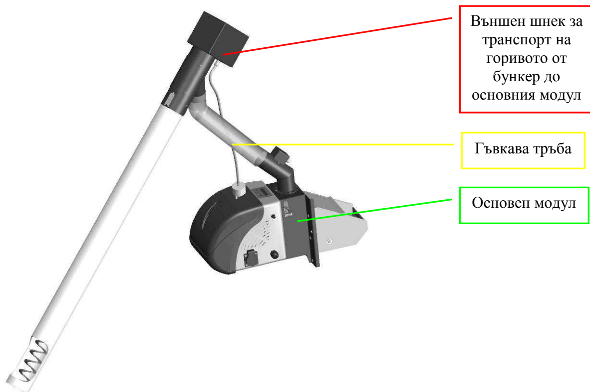
Фигура 2.3. Разположение на основните модули на пелетната горелка (поглед от страни);
