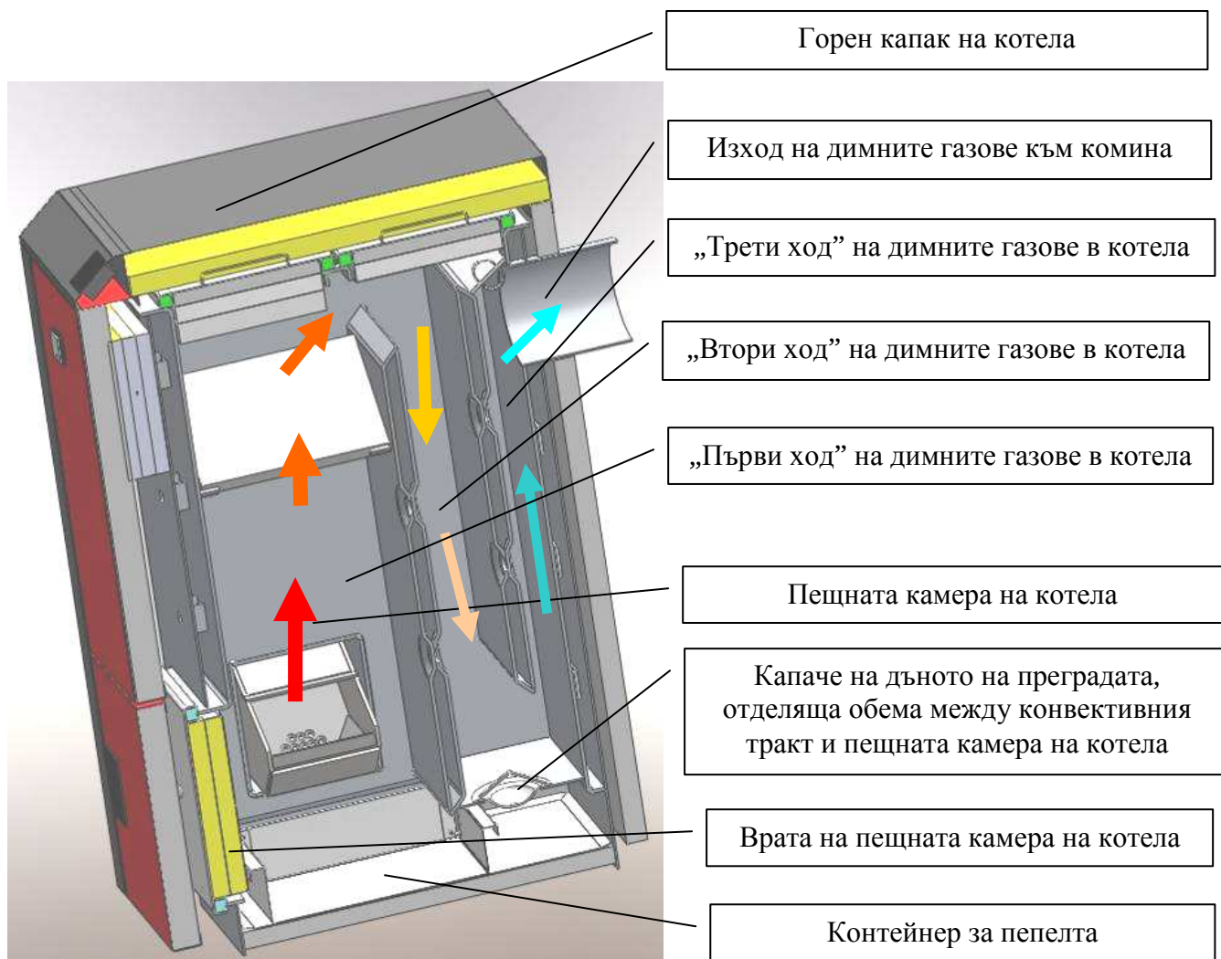
Фигура 3.6. Напречен разрез на пелетния водогреен котел от серията “Pelletherm v4” с посочен ход на димните газове и основни модули от конструкцията – (показан е вариант на системата с ляв монтаж на горелката);
