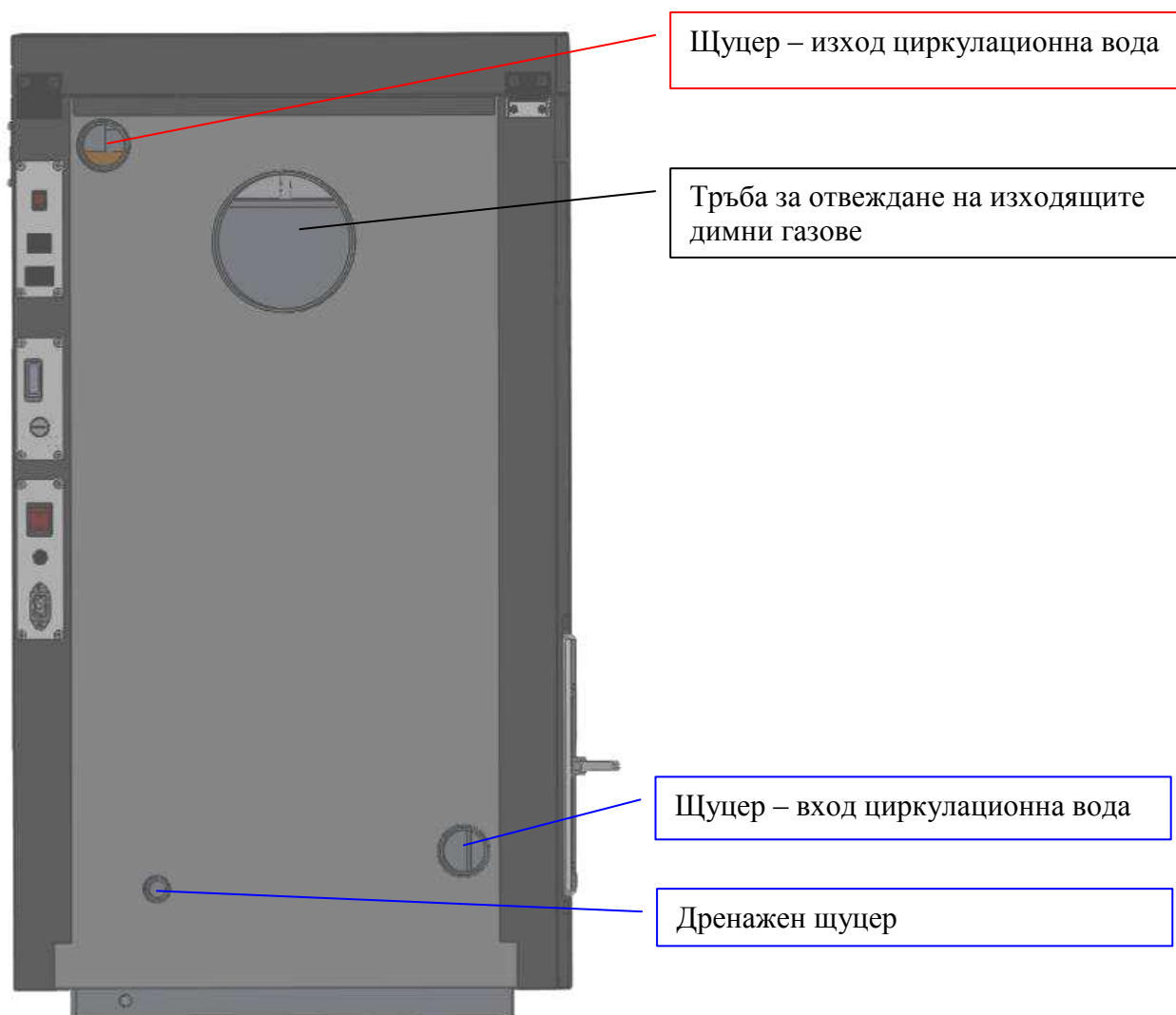
Фигура 4.1. Изглед към задната страна на водогрейния котел от серията “Pelletherm v4” ( показан е вариант с ляв монтаж на пелетната горелка );
