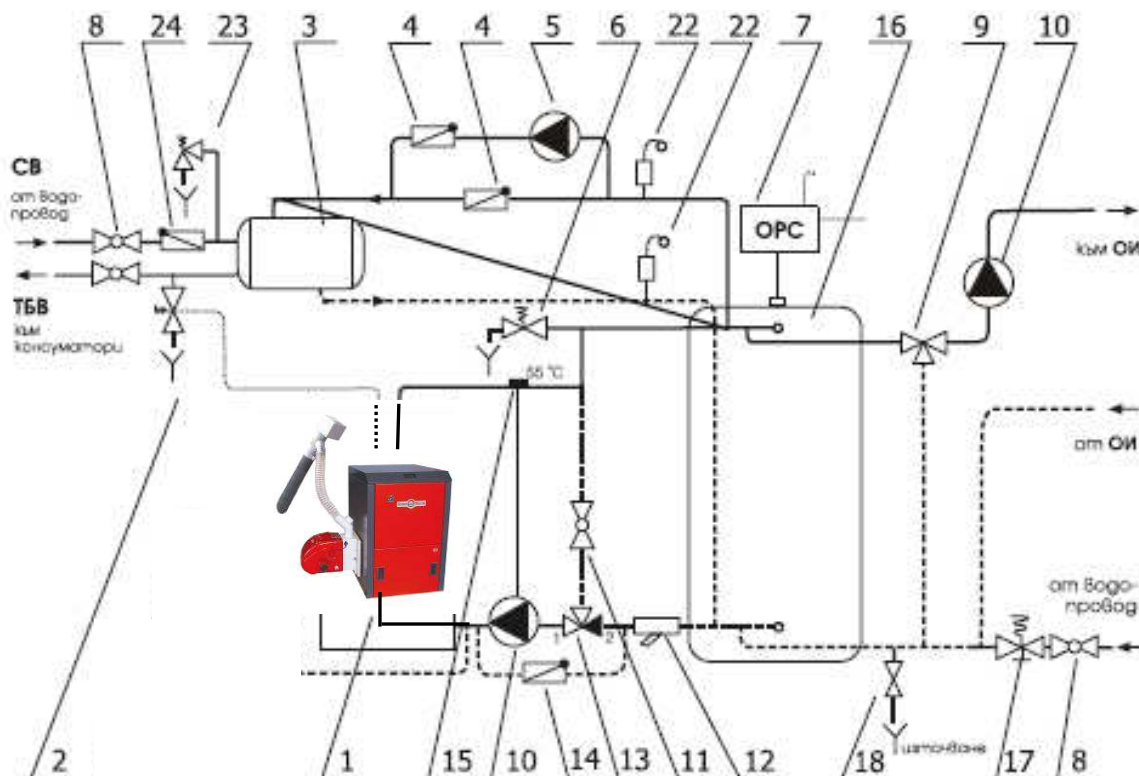
Фигура 4.13. Препоръчителна принципна хидравлична схема за свързване водогрейния котел от серията “Pelletherm v4” към отоплителна система, смесителен вентил и топлоакумулатор;
