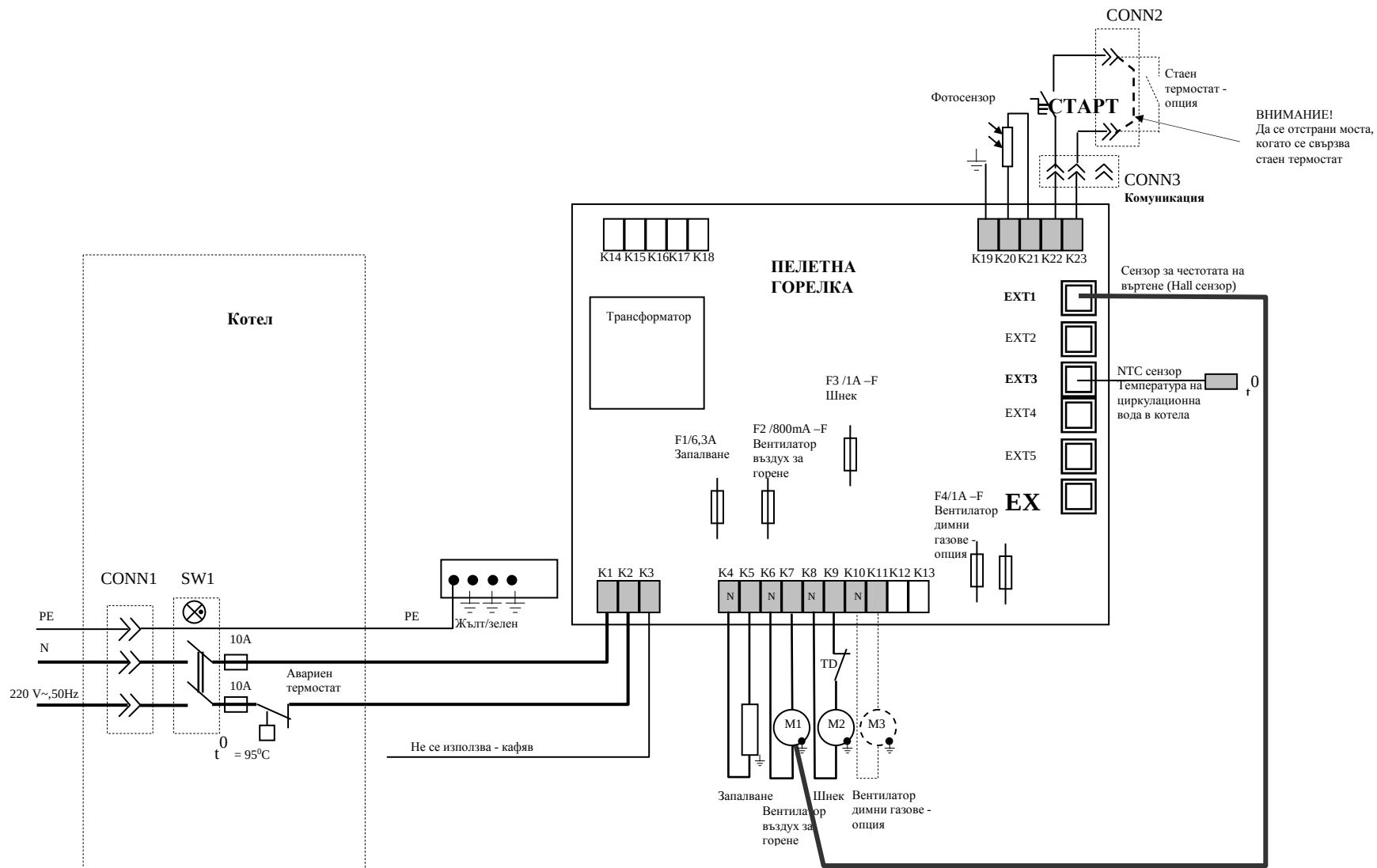
Фигура 6.1. Принципната електрическа схема на таблото за управление на водогрейния пелетен котел от серията „Pelletherm v4”, работещ в система с пелетна горелка от серията “GP IV”;
