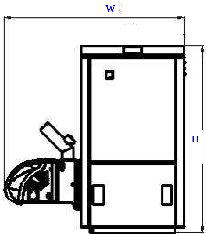
Фигура 3.1. Изглед на пелетен водогрееен котел от серията “Pelletherm v4” (с посочени габаритни размери) – поглед отпред;
