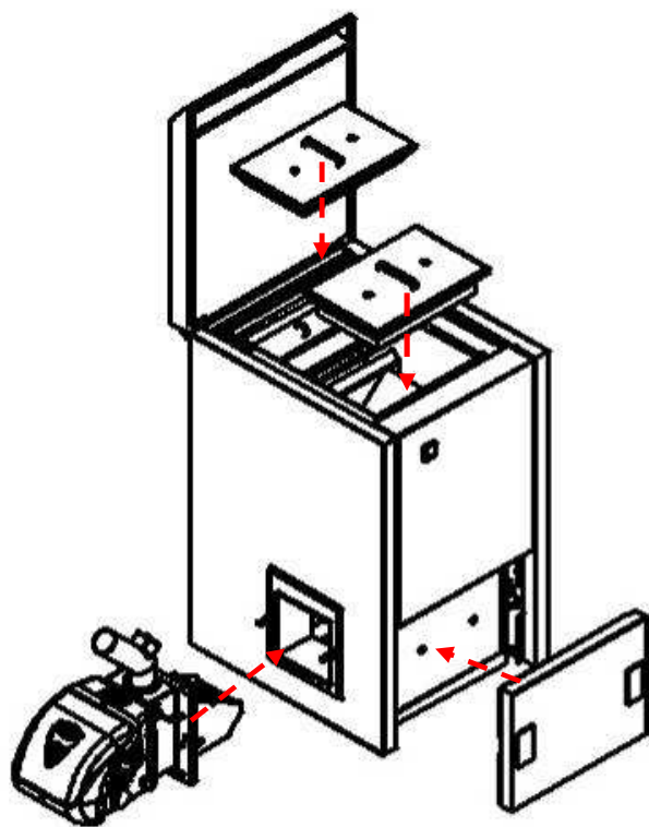
Фигура 4.8. Поставяне на капаци на пелетен котел от серията “Pelletherm v4”;
