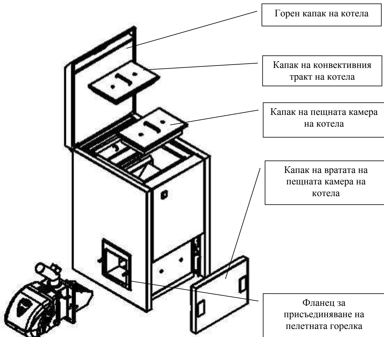
Фигура 3.5. Изглед на системата: пелетен водогрееен котел от серията “Pelletherm v4” и горелка за пелети от серията “GP IV” – (показан е вариант на системата с ляв монтаж на горелката);
