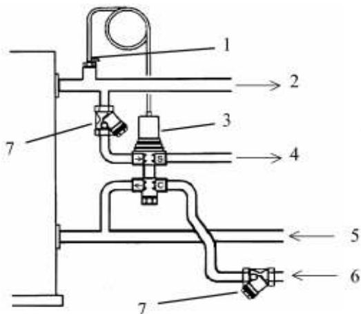
фиг. 8 Хидравлична схема
