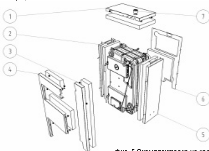
фиг. 5 Окомплектовка на котела
