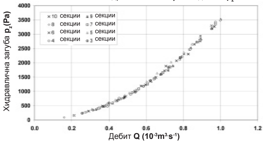
Фиг. 1 Хидравлична загуба на котелното тяло
