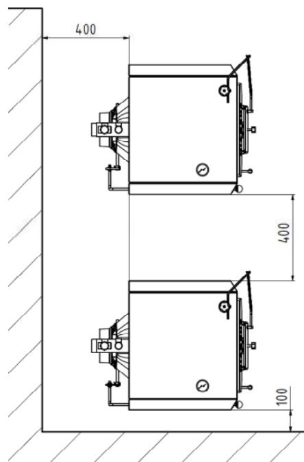
Фигура 10 Разположение на котлите в котелното помещение
