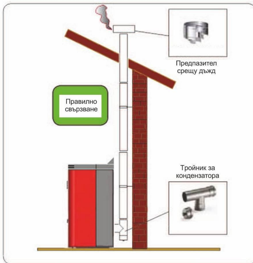
Фигура 3.2. Вътрешен монтаж на комина – правилно свързване.
