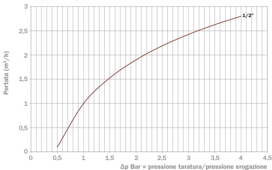
DIAGRAMMA PORTATE
